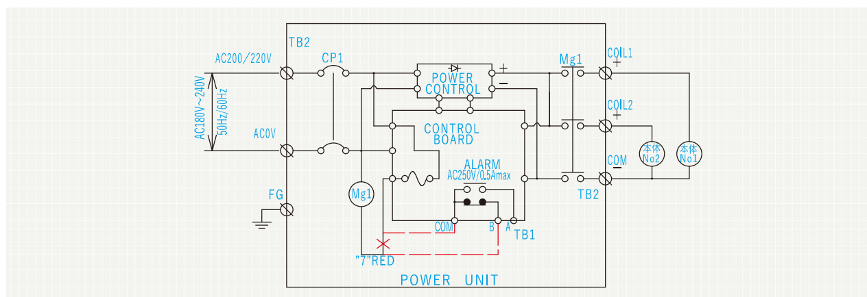
ブロック図 Block drawing
